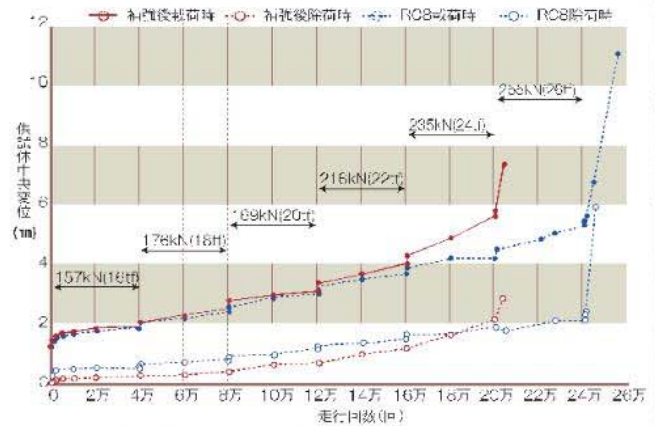
旧建設省土木研究所(現)土木研究センター、民間15社による共同研究「道路橋床版の輪荷重走行試験における疲労耐久性評価手法の開発」(平成11年10月)より
